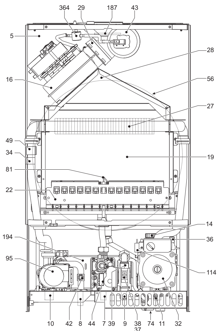
рис. 17 - Общий вид
