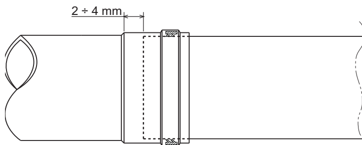
рис. 8 - Тепловое расширение
