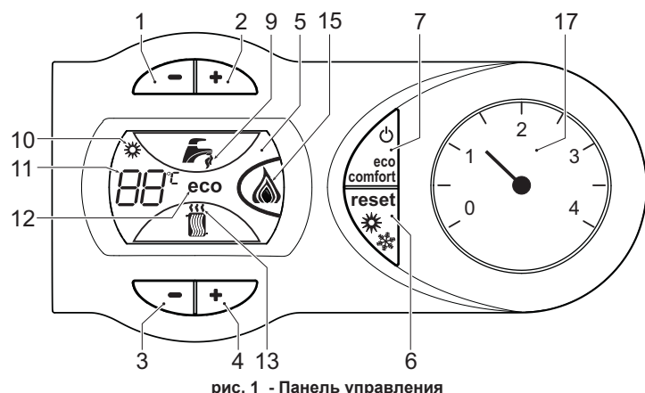
рис. 1 - Панель управления
