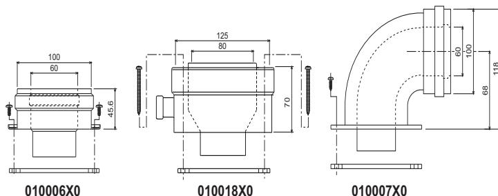
рис. 10 - Начальные элементы для коаксиальных воздуховодов
