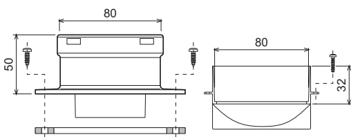
рис. 12 - Соединительный элемент для отдельных труб
